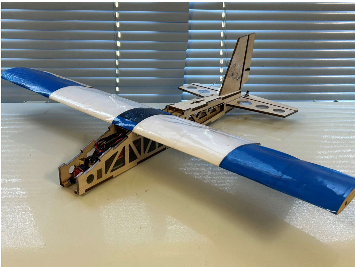
図 4 : 機体全貌
