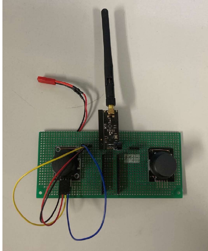
図 5 : 自作コントローラー
