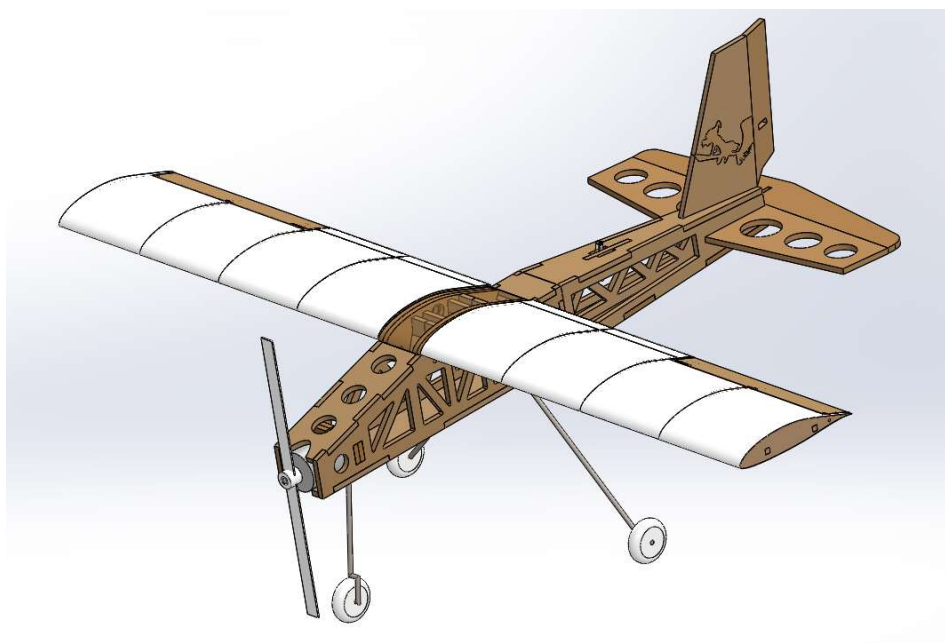
図 2：模型航空機の完成図
