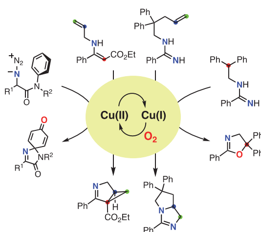
銅触媒による酸素酸化
