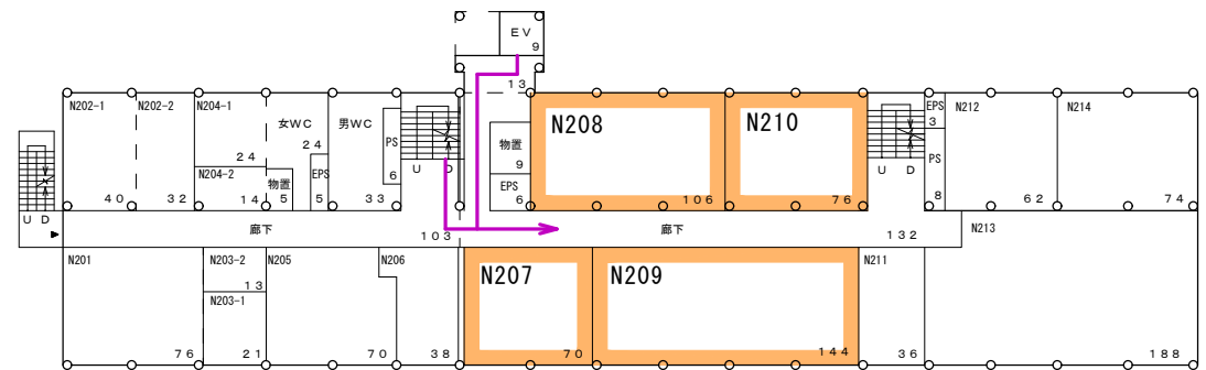
2階平面図
