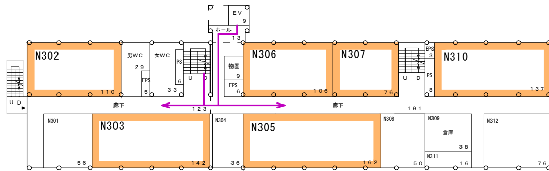
3階平面図
